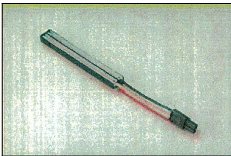
⑤プラス（赤コード）が左、マイナス（黒コード）が右になるように吹き抜いたピンで、端子に挿入します。
