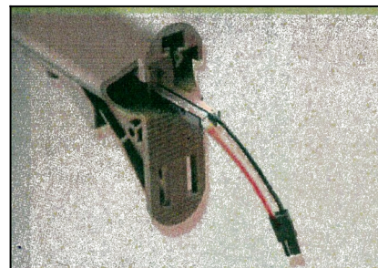
⑥ストック端子（金属面）が上になるようにストック内に入れます。
